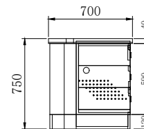
左右视图
