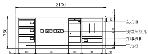
主视图
