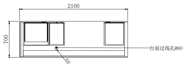
俯视图
